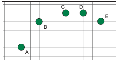
3.16 Stroboskopbild
