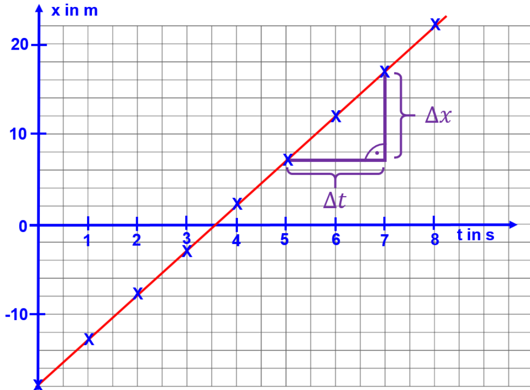
Abb. 4: x - t -Diagramm
