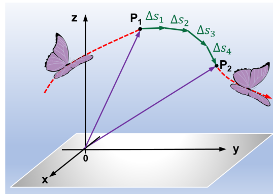
Abb. 8: Wegelemente und Gesamtweg
