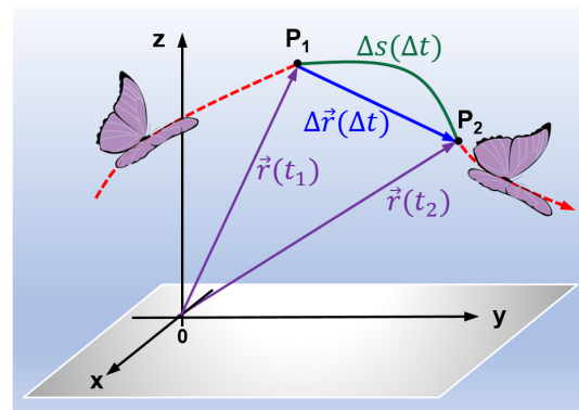
Abb. 7: Ortsverschiebung u. Wegelement
