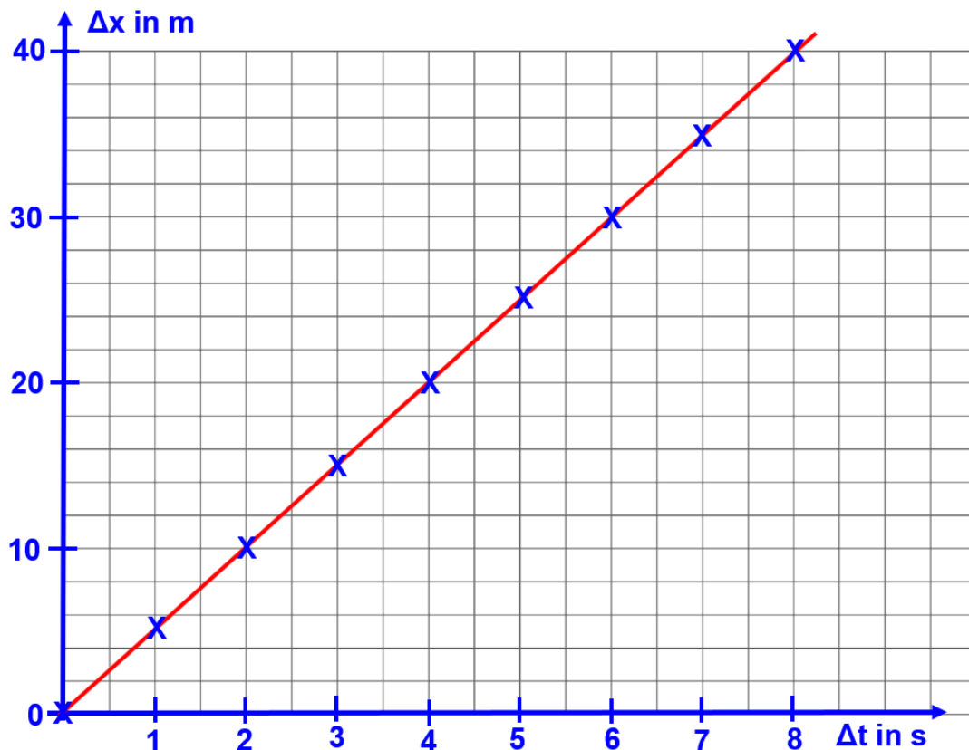
Abb. 5: \Delta x - \Delta t -Diagramm
